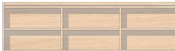
Triple Open Wall Unit H341 H490 x W1555 x D285mm H19¼ x W61¼ x D11¼ inches
