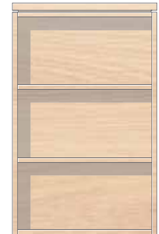
Tall Open Wall Unit H145 H950 x W520 x D285mm H37½ x W20½ x D11¼ inches
